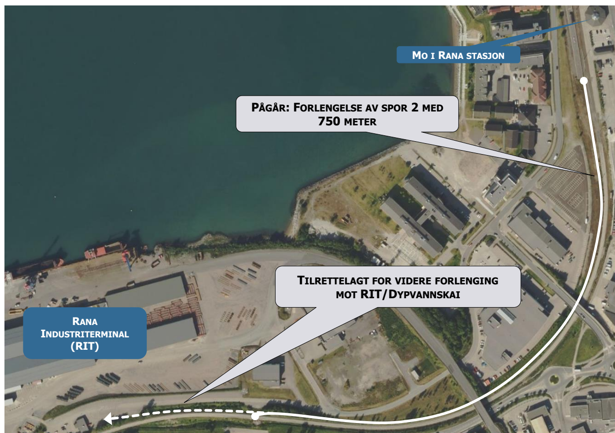
Figur 3-13: Forlengelse av kryssingsspor Mo i Rana stasjon
